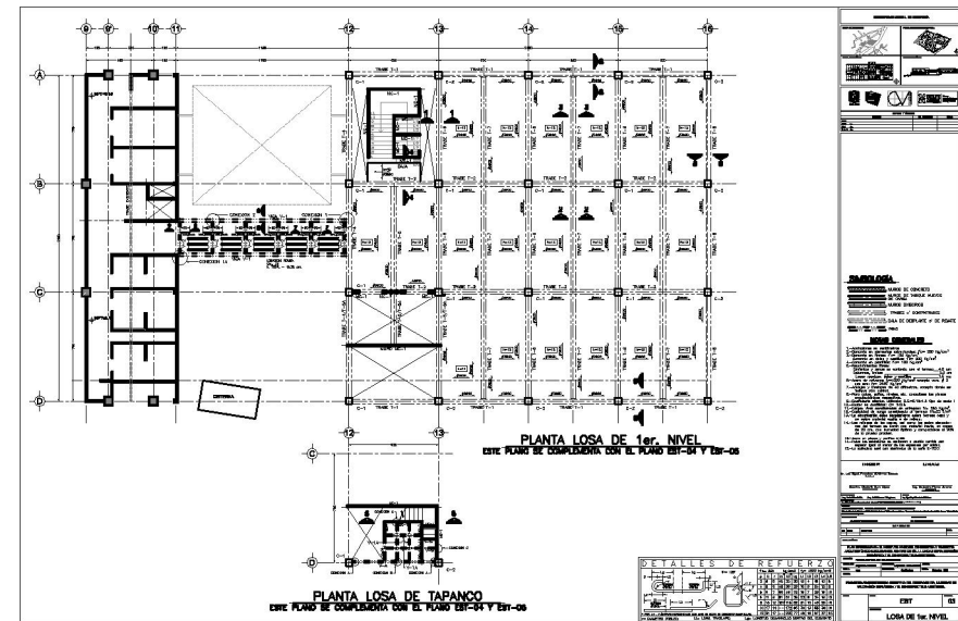
Planta estructural
