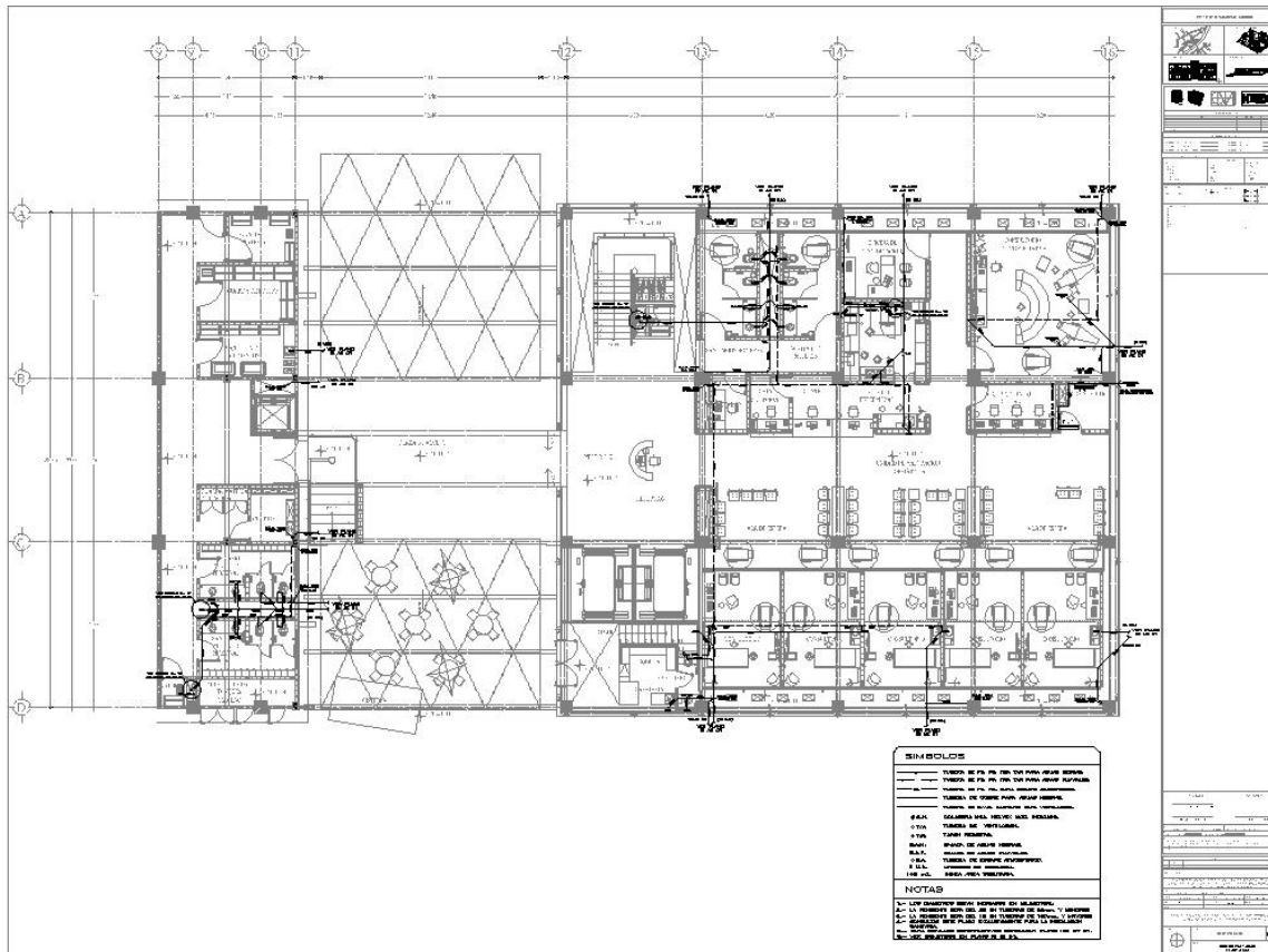
Instalación de Gas – Tuberías
