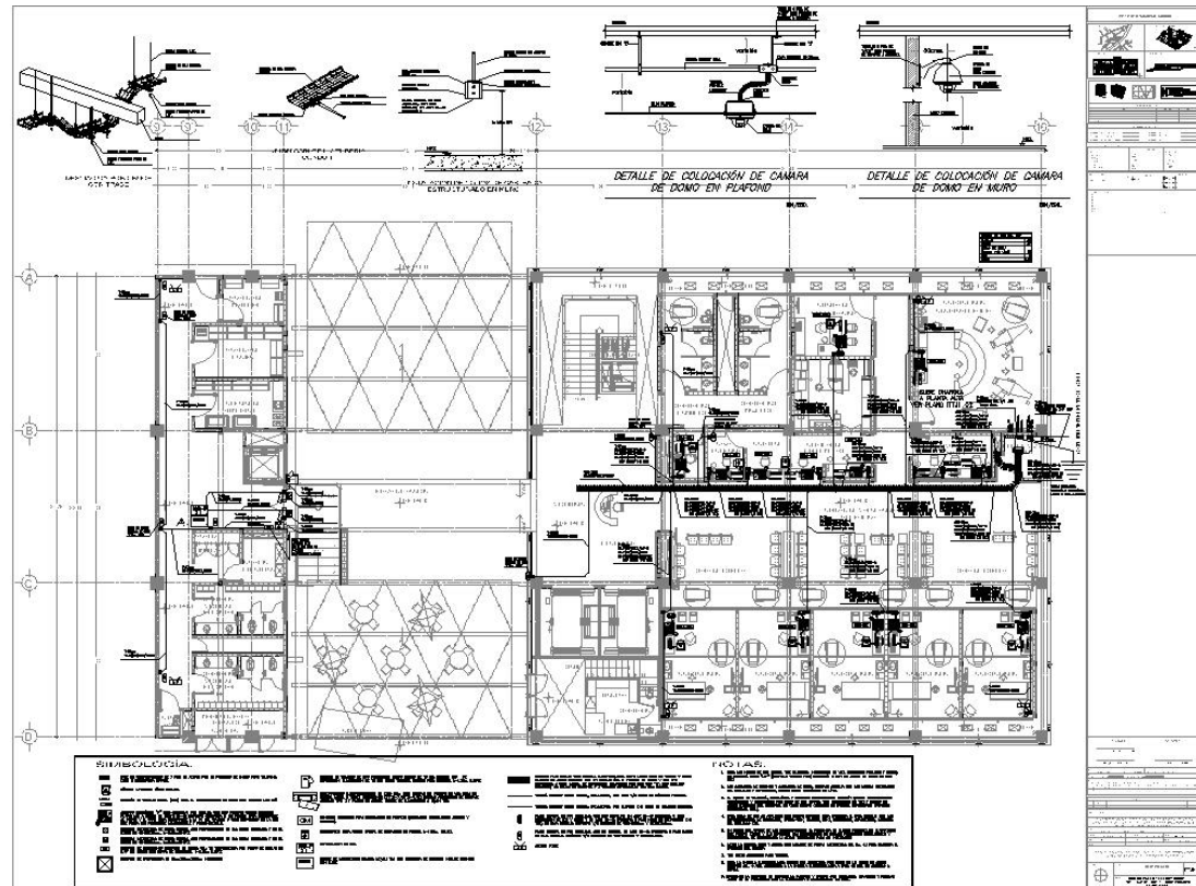
Planta Instalación de Voz y Datos
