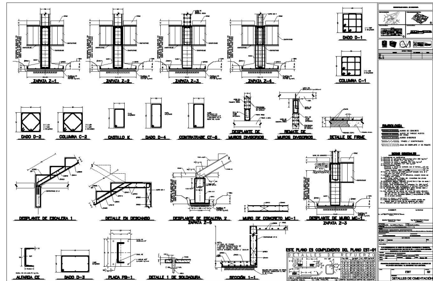
Detalles de cimentación
