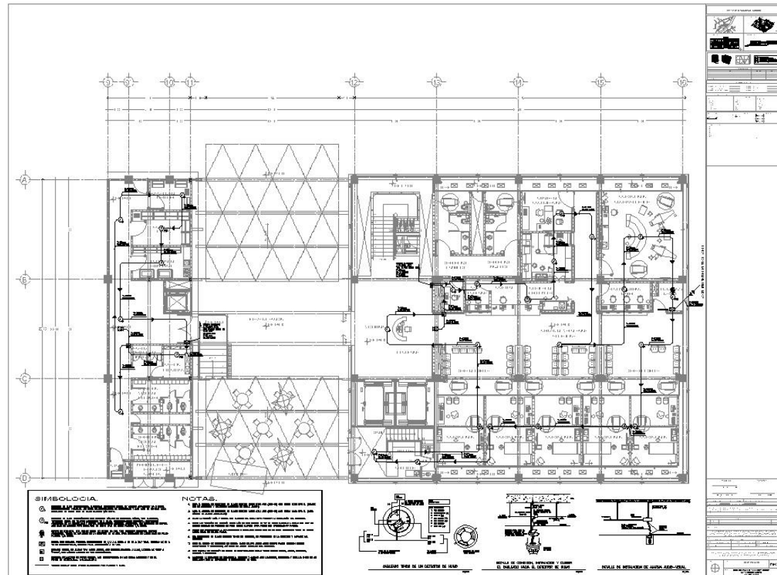
Planta de sistema de detección contra-incendios
