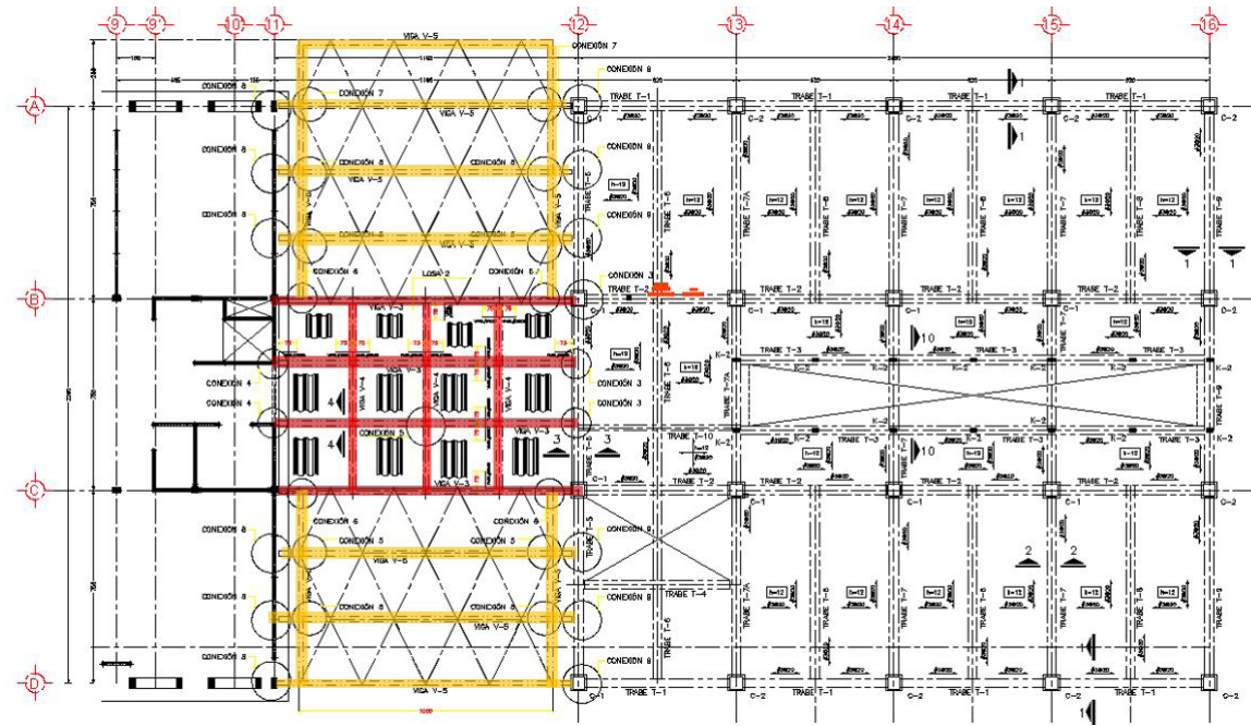
Ejemplo de generador de estructuras- secciones de acero estructural
