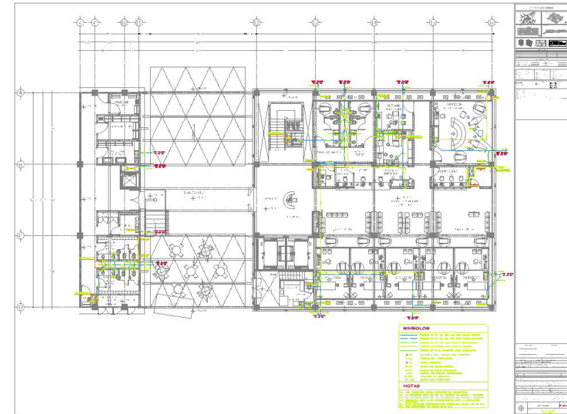
Planta Instalación sanitaria
