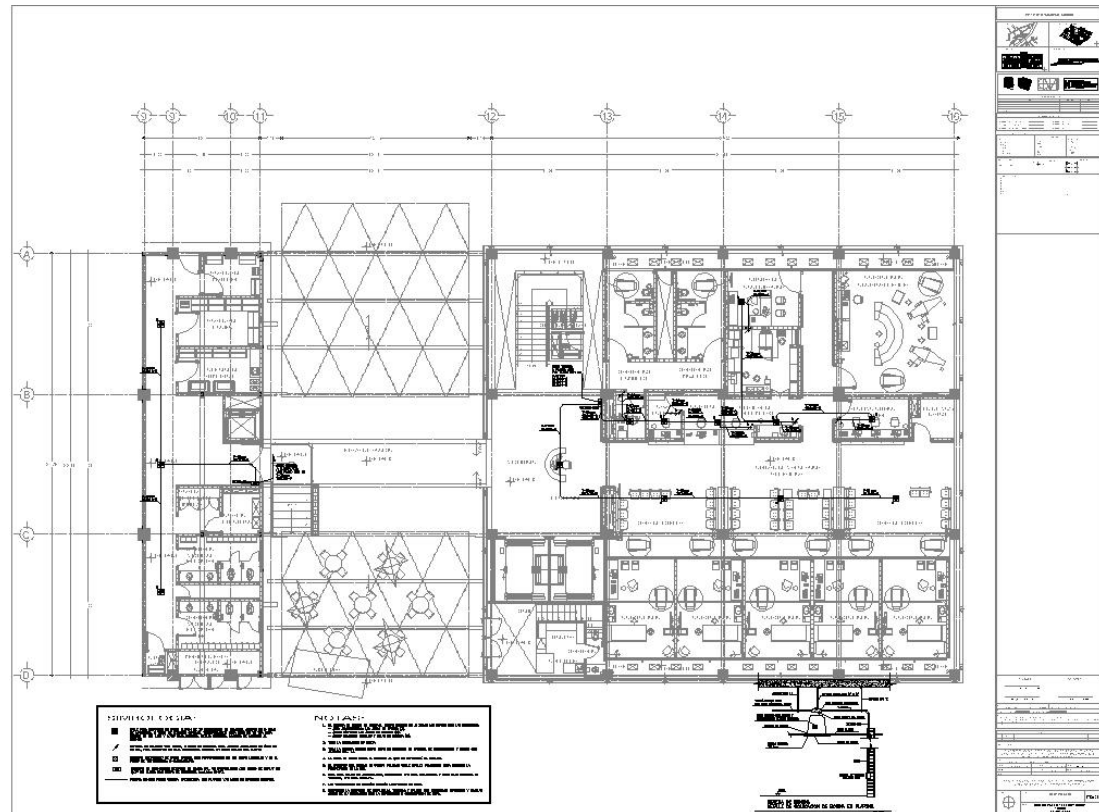
Planta Instalaciones de comunicación
